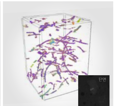
합성섬유(폴리프로필렌) 콘크리트 분산도 Test [ 분산도 우수하나, 재료 물성치 불량 ]
